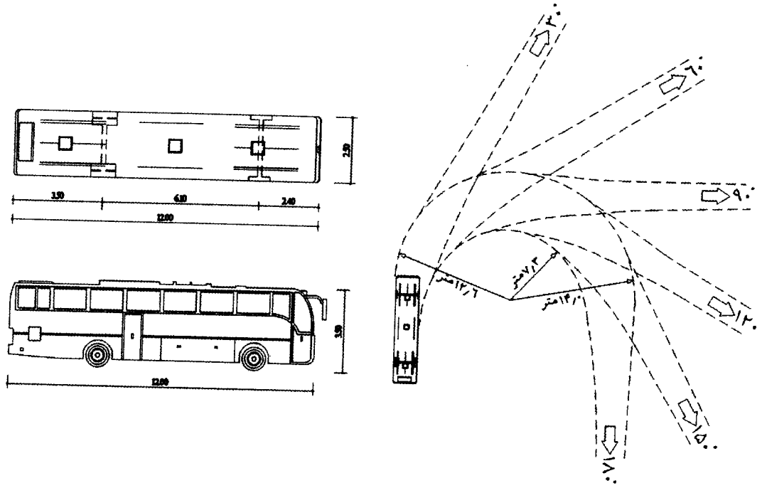
شکل ۳-۶: ابعاد و مسیر گردش اتوبوس تیب
