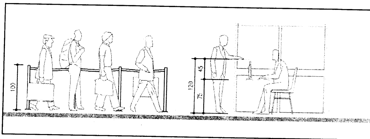
شکل ۶-۲: غرفه فروش بلیت
